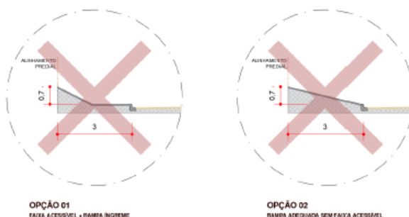
Figura 4 – Opções inadequadas de execução da calçada devido ao desnível
