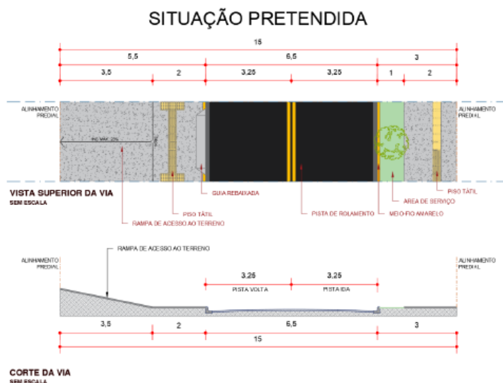
Figura 5 – Solução da calçada para acesso aos terrenos com desnível relevante
